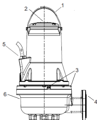
Рис. 1 Насос FK
