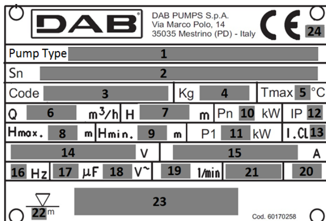
Afb. 3 Typeplaatje
