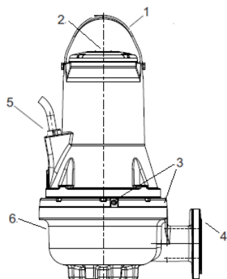
Fig. 1 Pompa FK
