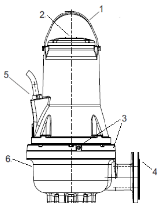
Rys. 1 Pompa FK
