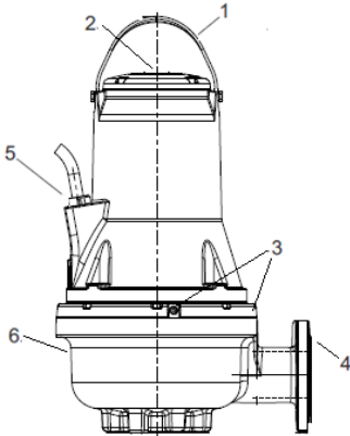
Şekil 1 FK pompası
