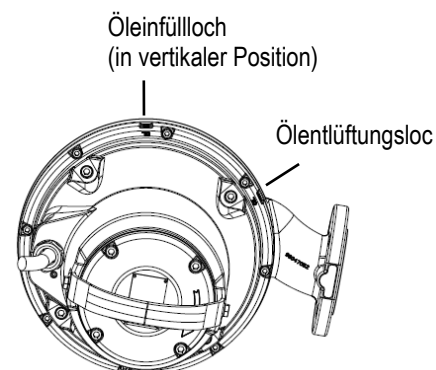
Abb. 11 Öleinfüllöffnungen
