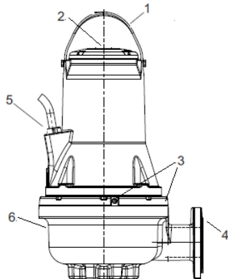
Fig. 1 Bomba FK
