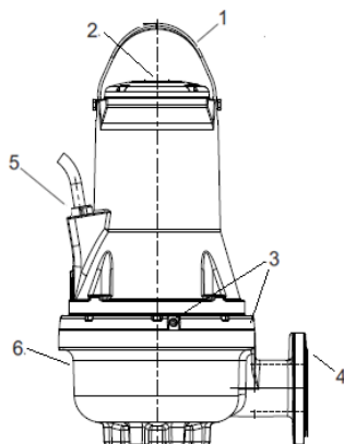
Slika 1 FK črpalka
