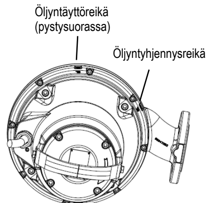
Kuva 11 Öljyn täyttöaukot
