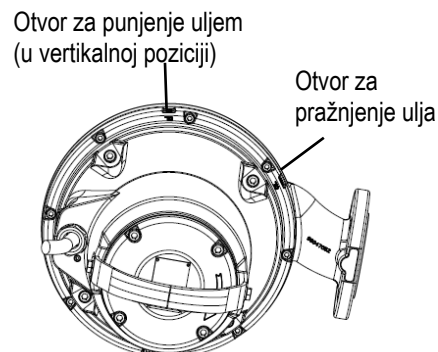
Slika 11 Punjenje uljem
