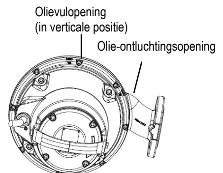
Afb. 11 Olievulopeningen
