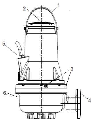
Slika 1 FK crpka
