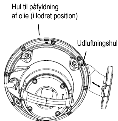
Fig. 11 Oliepåfyldningshuller
