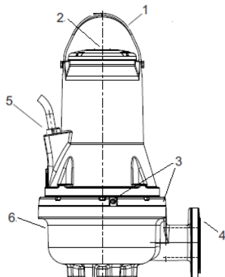
Fig. 1 Pompe FK
