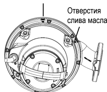
Рис. 11 Маслоналивные отверстия
